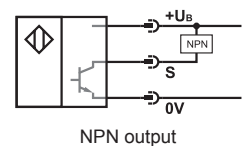
NPN output
