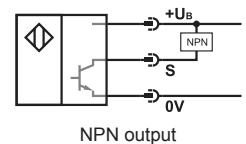
NPN output
