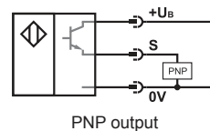
PNP output
